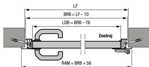
Stranska vrata z aluminijastim kotnim vratnim okvirjem profil tipa 1 ali 2 Pritrditev na notranji strani
