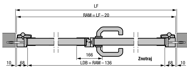
2-krilna stranska vrata z aluminijastim fiksnim vratnim okvirjem profil tipa 2 Vgradnja v odprtino
