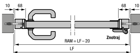
Stranska vrata z aluminijastim fiksnim vratnim okvirjem profil tipa 2 Vgradnja v odprtino
