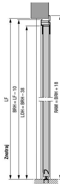
Stranska vrata z aluminijastim kotnim vratnim okvirjem profil tipa 2 Zunanji prislon
