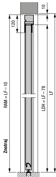
Stranska vrata z aluminijastim fiksnim vratnim okvirjem profil tipa 2 Vgradnja v odprtino
