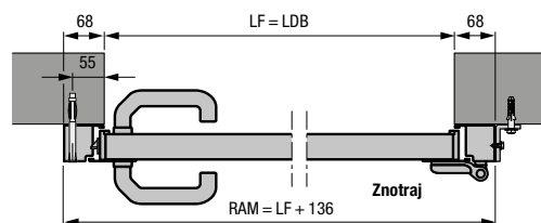
Stranska vrata z aluminijastim fiksnim vratnim okvirjem profil tipa 1 Vgradnja za odprtino
