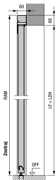
Stranska vrata z aluminijastim fiksnim vratnim okvirjem profil tipa 2 Vgradnja za odprtino
