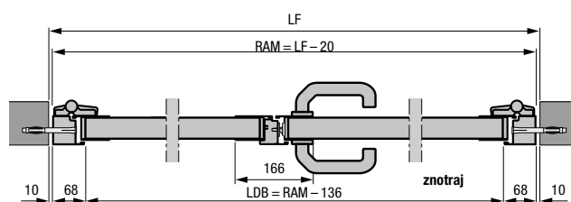
2-krilna stranska vrata z aluminijastim slepim okvirjem tip profila 2 vgradnja v odprtino
