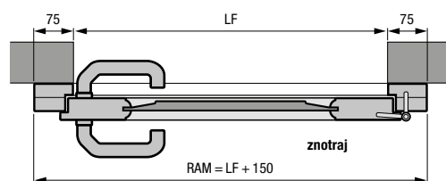
Stranska vrata iz masivnega lesa vgradnja za odprtino
