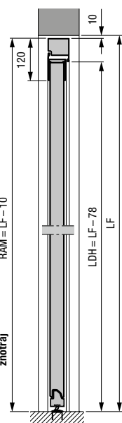
Stranska vrata z aluminijastim slepim okvirjem tip profila 2 vgradnja v odprtino
