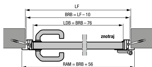
Stranska vrata z aluminijastim kotnim okvirjem tip profila 1 ali 2 Notranji prislon
