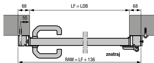
Stranska vrata z aluminijastim slepim okvirjem tip profila 1 vgradnja za odprtino
