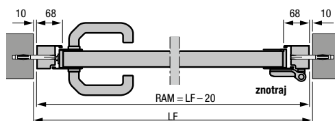
Stranska vrata z aluminijastim slepim okvirjem tip profila 2 vgradnja v odprtino
