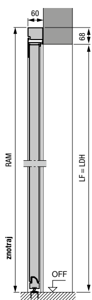
Stranska vrata z aluminijastim slepim okvirjem tip profila 2 vgradnja za odprtino
