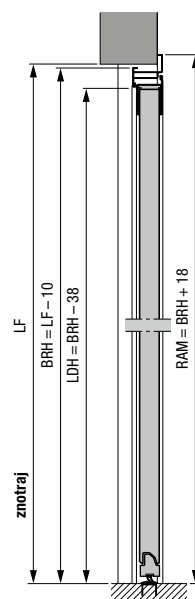
Stranska vrata z aluminijastim kotnim okvirjem tip profila 2 Zunanji prislon
