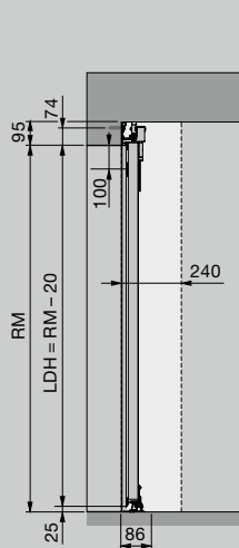
Stenska montaža kot drsna vrata
