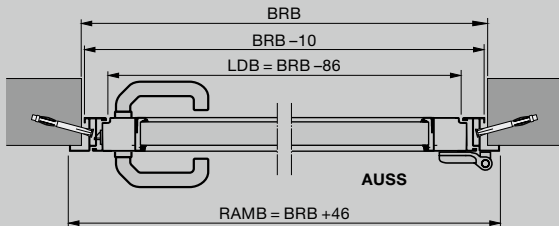
Stranska vrata s kotnim podbojem vgradnja pred odprtino
