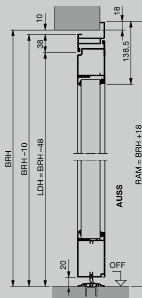
Stranska vrata z aluminijastim kotnim podbojem pritrditev na zunanji strani
