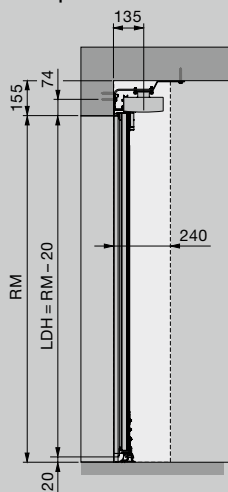
Stropna montaža B kot drsna vrata
