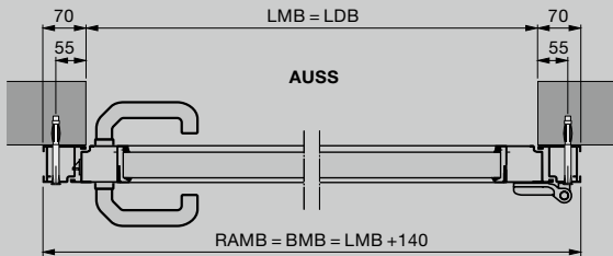
Stranska vrata z aluminijastim slepim podbojem vgradnja za odprtino
