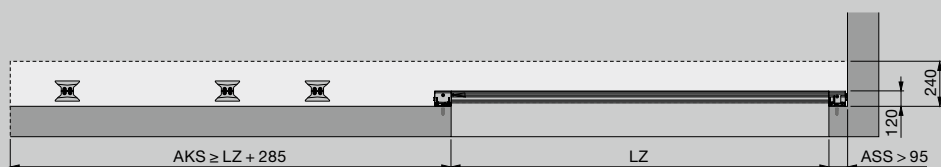
Stenska montaža kot drsna vrata (rezanje talnega vodila)
