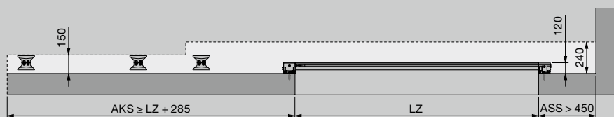
Stropna montaža B kot drsna vrata (rezanje talnega vodila)
