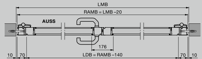
2-krilna stranska vrata z aluminijastim slepim podbojem vgradnja v odprtino
