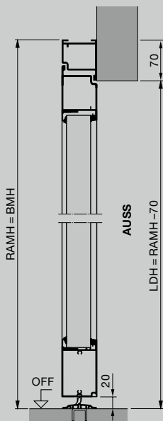
Stranska vrata z aluminijastim slepim podbojem vgradnja za odprtino
