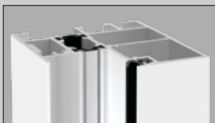
Pravokotna izvedba (profil A2)
