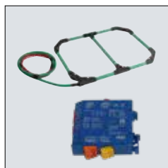
Detektor indukcijske zanke in končna indukcijska zanka
