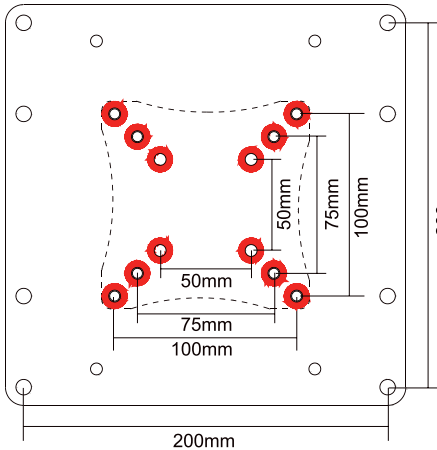
Fig.2: innere VESA-Lochabstände
