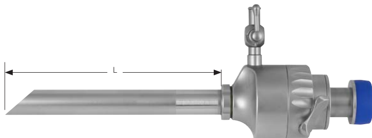
Automatik Trokarhülse mit manueller Klappenöffnung Automatic trocar sleeve with multifunctional valve
