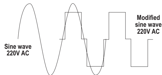
Fig. 1: AC Output
