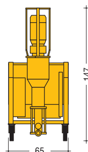
DIMENSIONES (cm)
