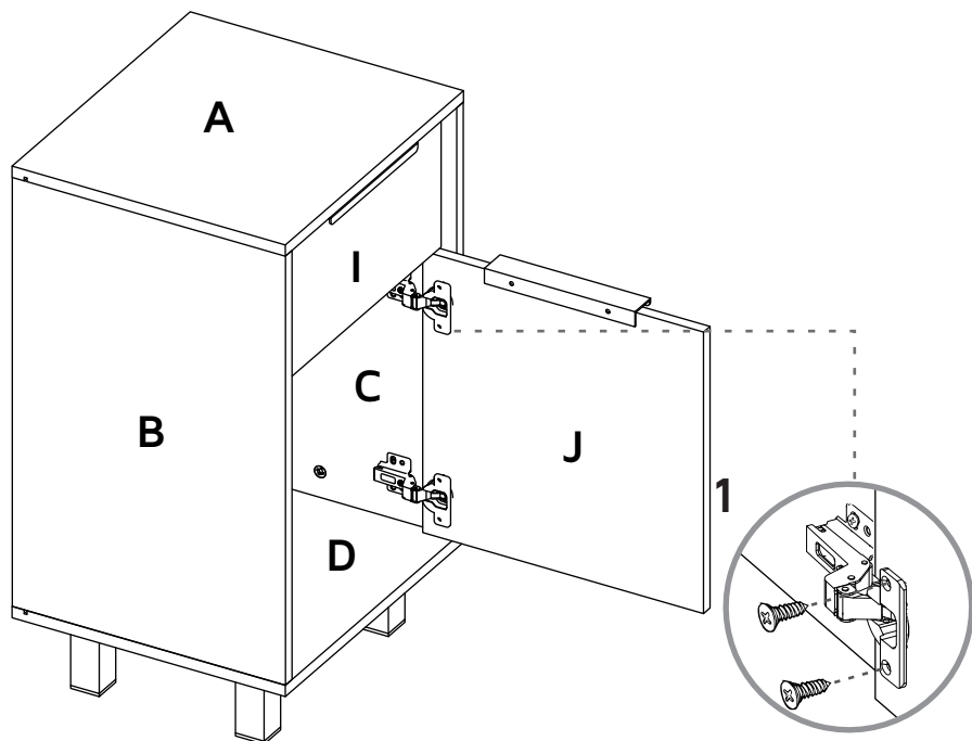
Ajuste de las bisagras Hinge adjustment
