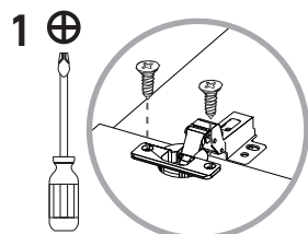
Ajuste de las bisagras Hinge adjustment
