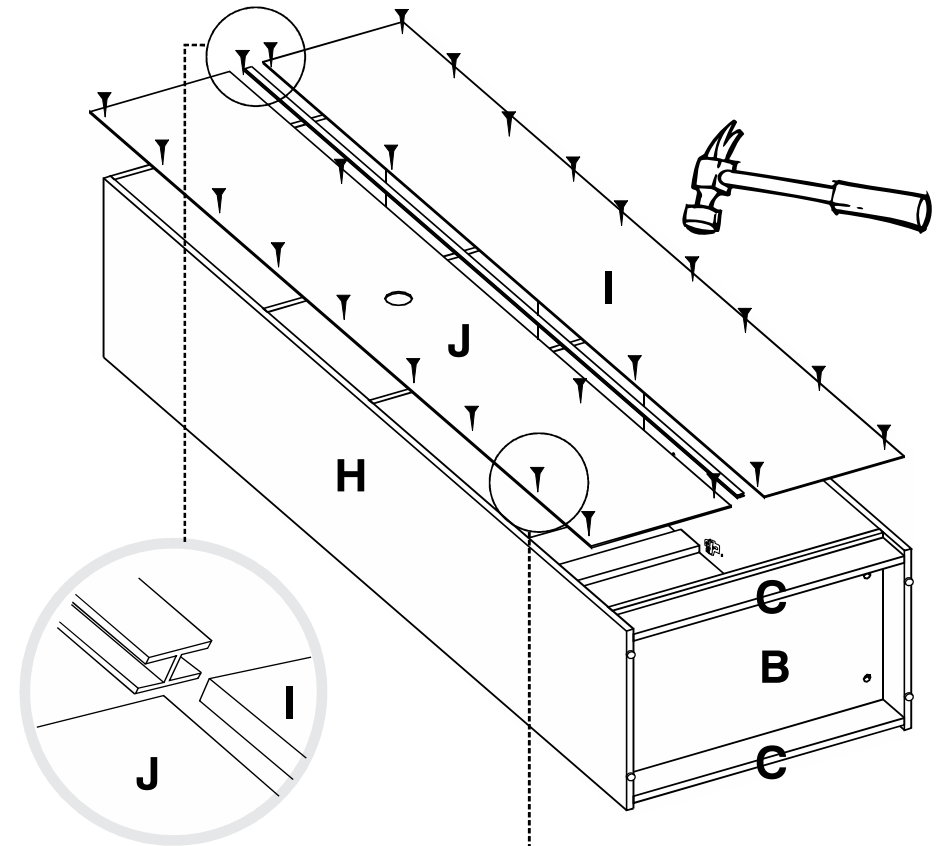
Perfil en H/ H Guide
