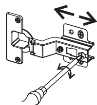
Ajuste de profundidad Depth adjustment
