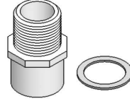
Adaptador macho PVC 1" con empaque de caucho de 1" por fuera (REBOSE).
