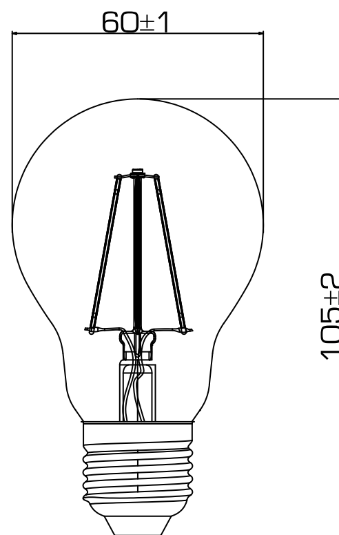
GRÁFICO CON DIMENSIONES (en mm)
