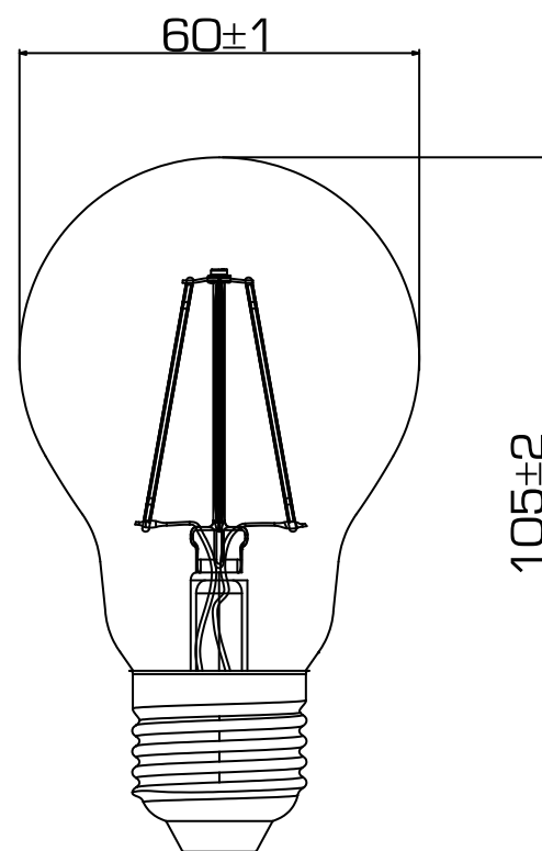
GRÁFICO CON DIMENSIONES (en mm)
