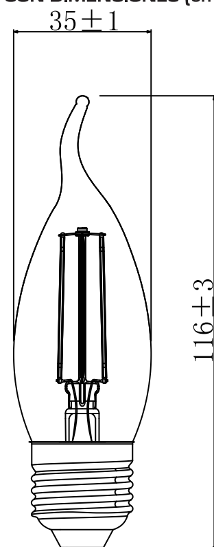
GRÁFICO CON DIMENSIONES (en mm)
