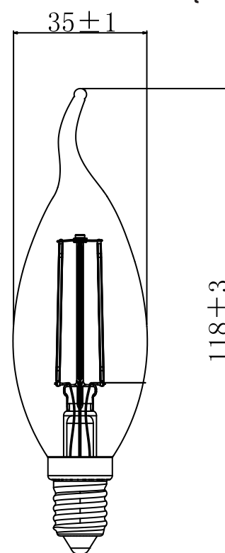
GRÁFICO CON DIMENSIONES (en mm)
