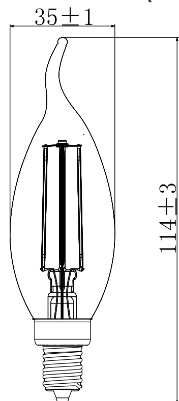
GRÁFICO CON DIMENSIONES (en mm)
