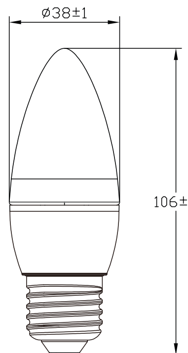
GRÁFICO CON DIMENSIONES (en mm)
