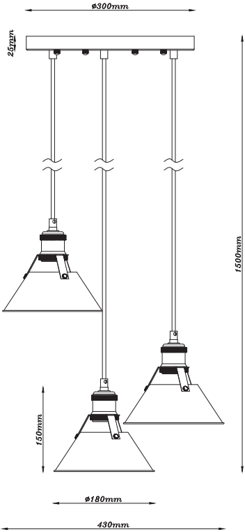
GRÁFICO CON DIMENSIONES (en mm)
