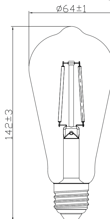
GRÁFICO CON DIMENSIONES (en mm)
