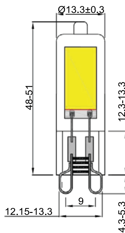
GRÁFICO CON DIMENSIONES (en mm)
