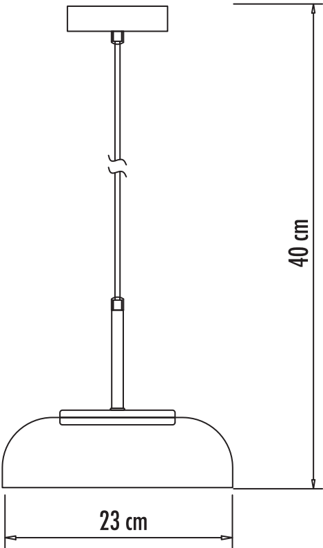
GRÁFICO CON DIMENSIONES
