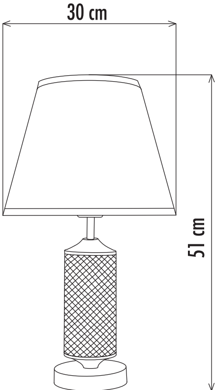
GRÁFICO CON DIMENSIONES
