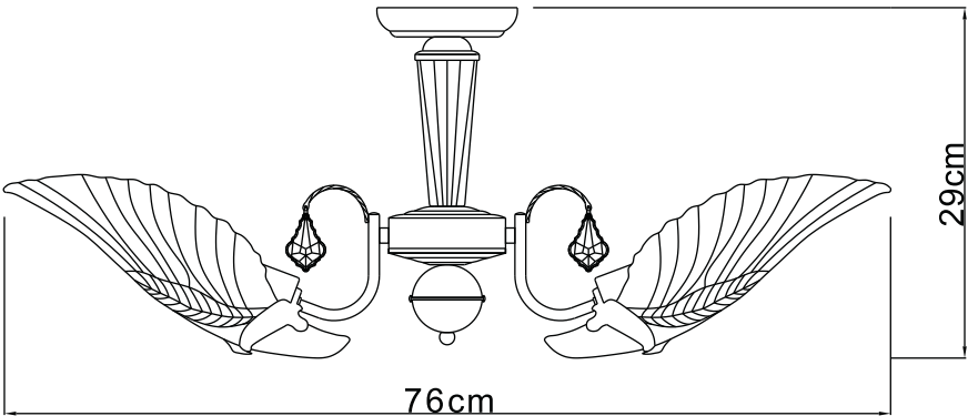
GRÁFICO CON DIMENSIONES
