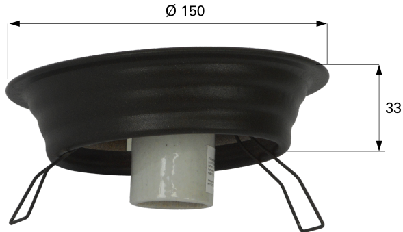
Medidas Aproximadas en mm
