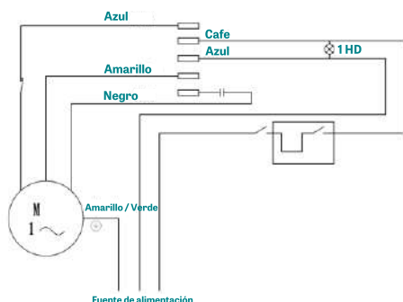
Bomba Presurizadora G2 y G3
