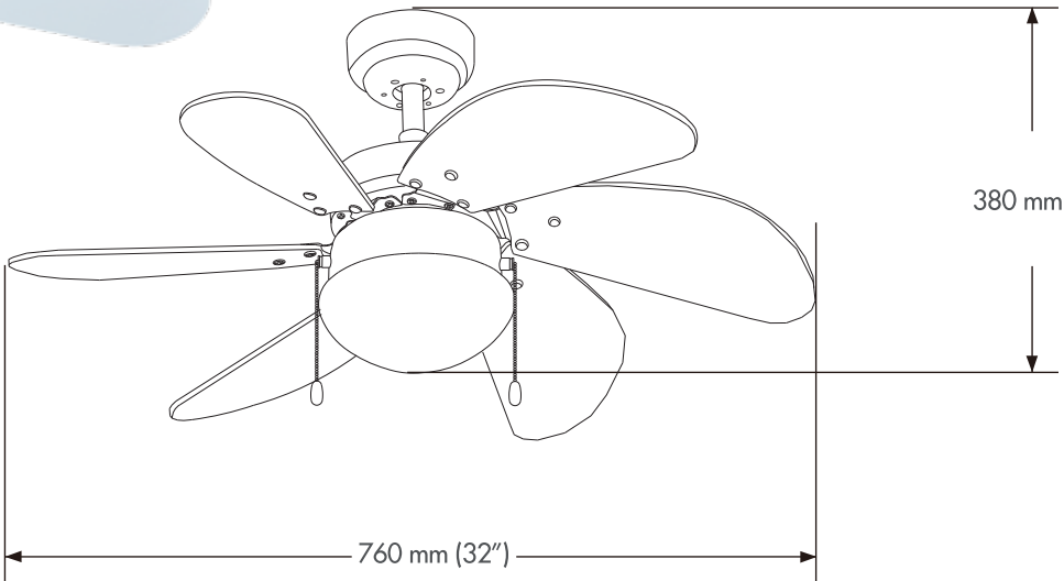
GRÁFICO CON DIMENSIONES
