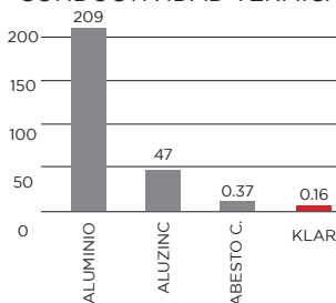
CONDUCTIVIDAD TÉRMICA
