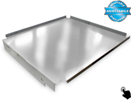
VE6215 Bianchi ITA Pianale base interno in acciaio inox 430 spessore 0,8mm 655x610mm adattabile per distributore automatico Lei 400 Lei 600 ENG Internal base plate in 430 stainless steel thickness 0,8mm 655x610mm adaptable for vending machine Lei 400 Lei 600
