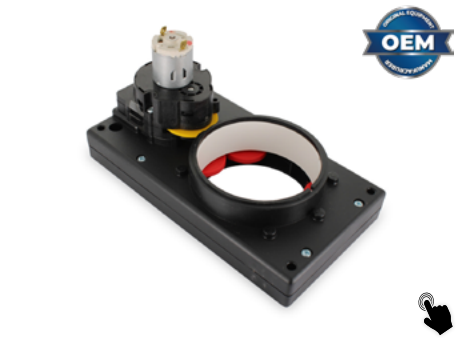
VE4030031100 4030031100 - 403.00.311.00 Sielaff ITA Separatore di tazze da 70 mm ENG 70mm cup separator
