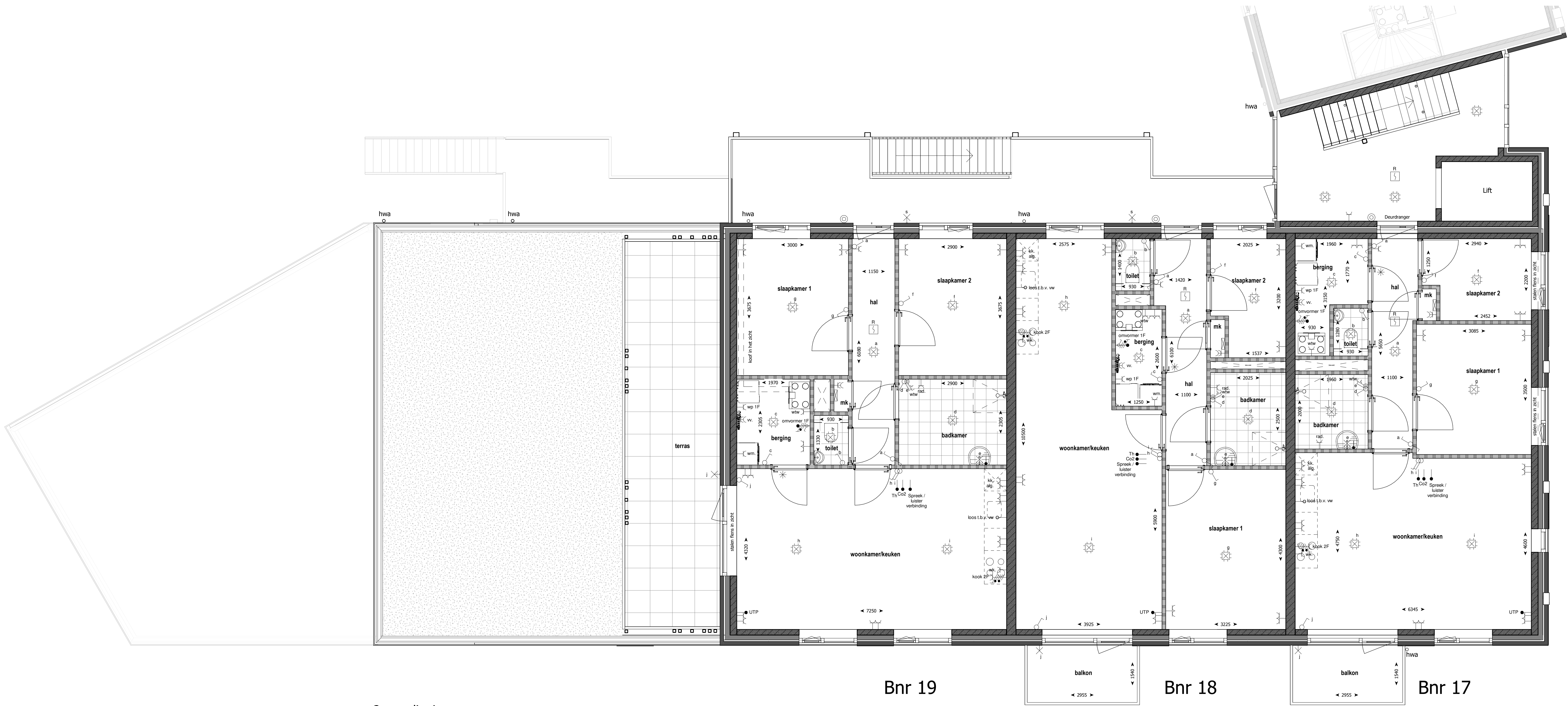
2e verdieping
