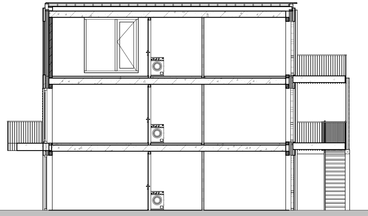
Doorsnede
