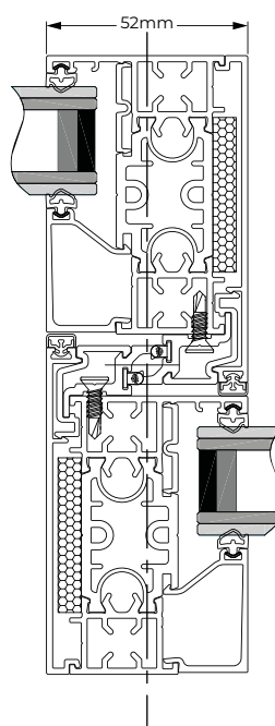
Slim Interlock
