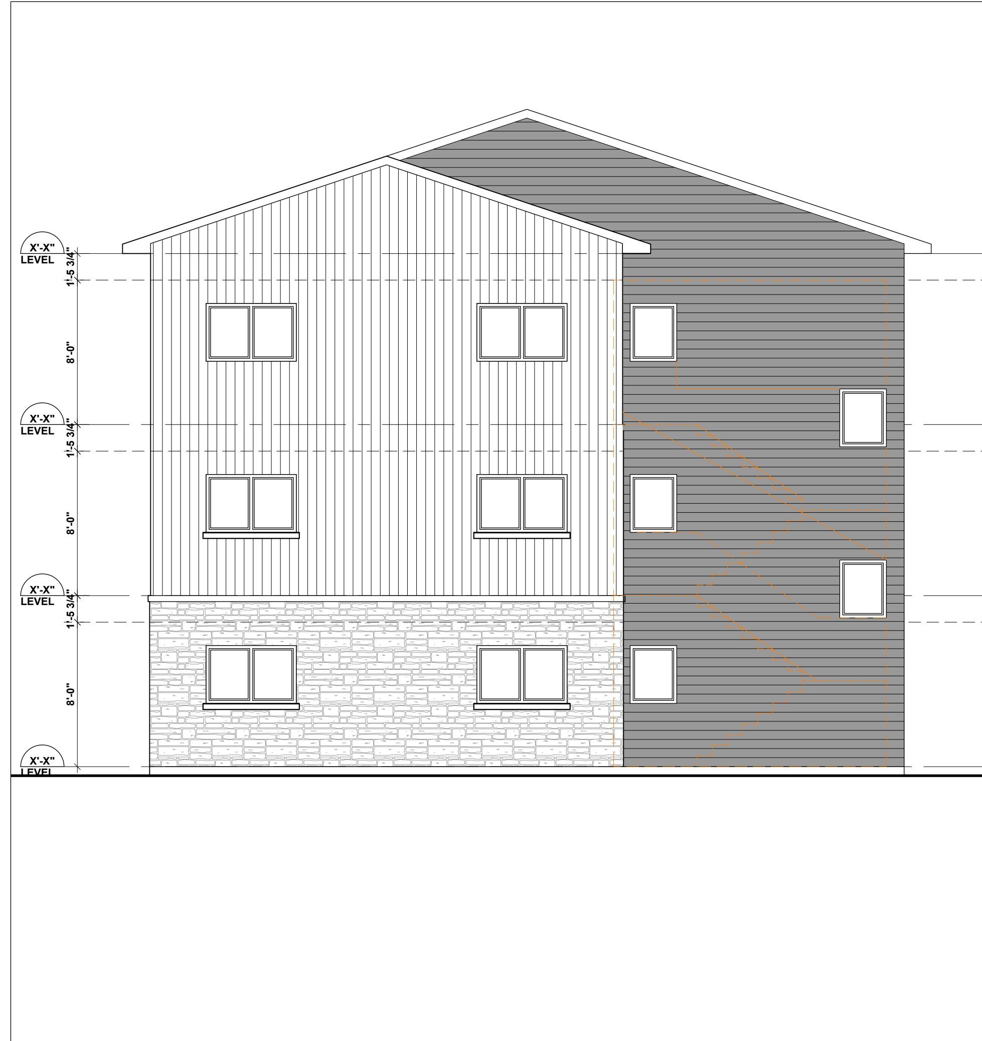
1 VIEWPORT TITLE A2008 SCALE: XX"=1'-0"
