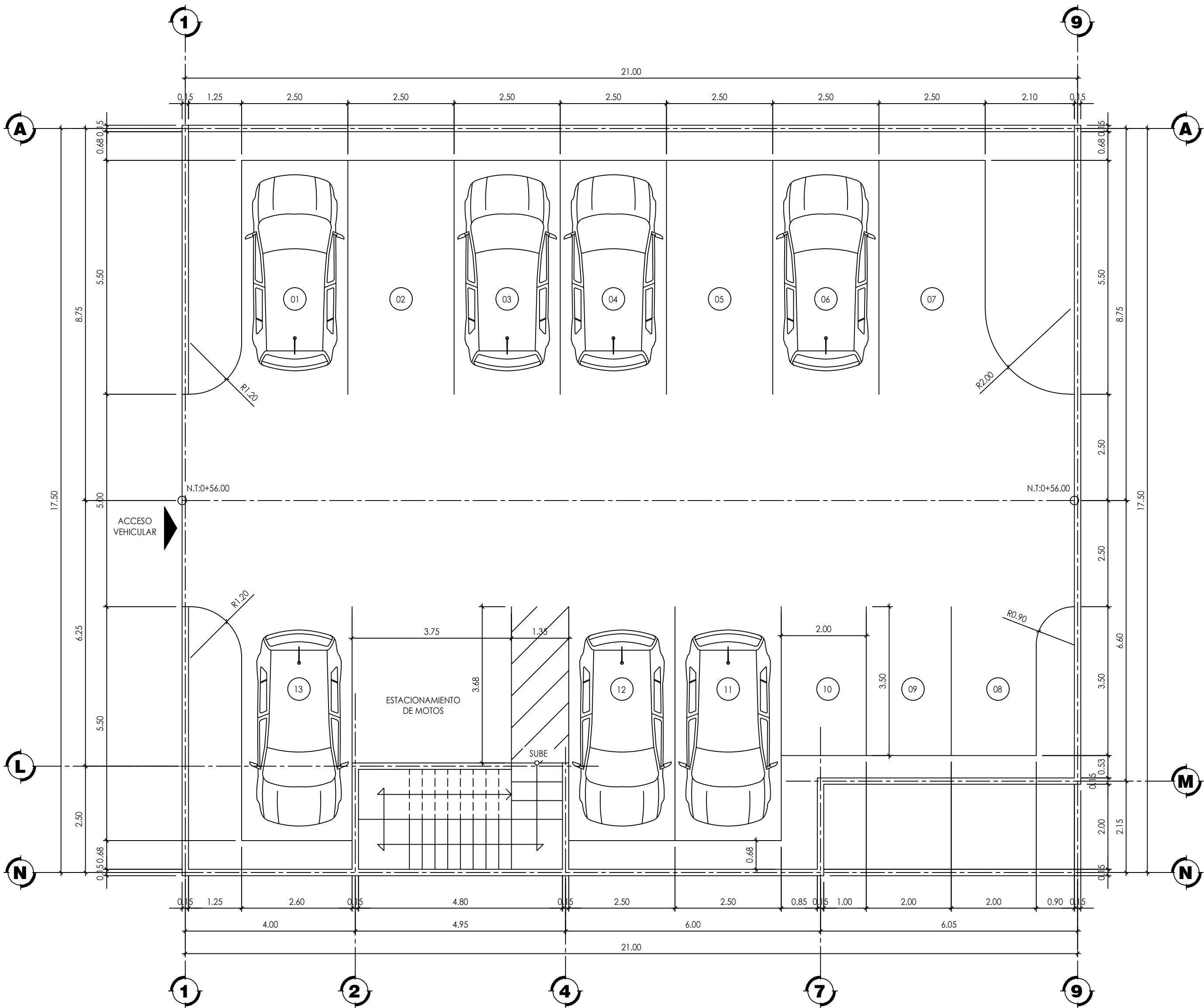
PLANTA ARQUITECTONICA ESTACIONAMIENTO SOTANO N:+56.00 ESC. 1:75
