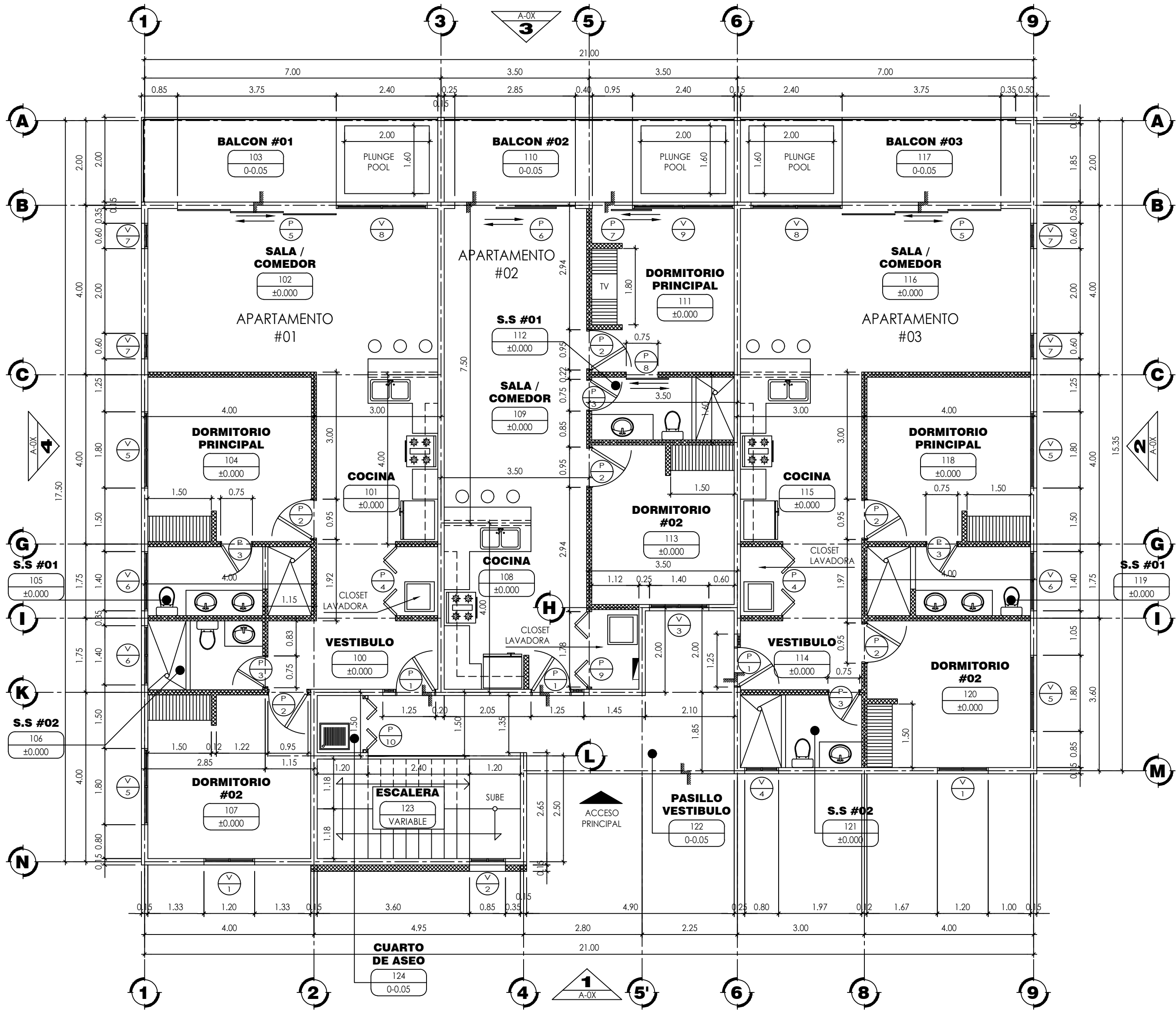
PLANTA ARQUITECTONICA PRIMER NIVEL N:+59.00 ESC. 1:75
