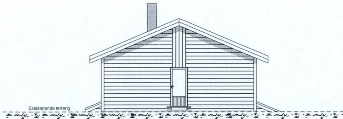
Fasade Øst
