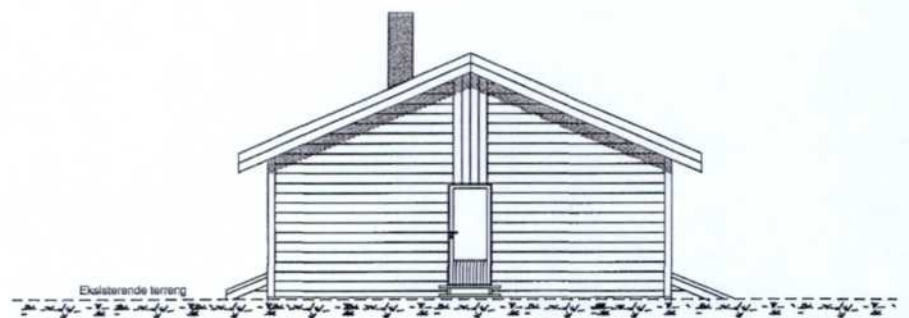
Fasade Øst
