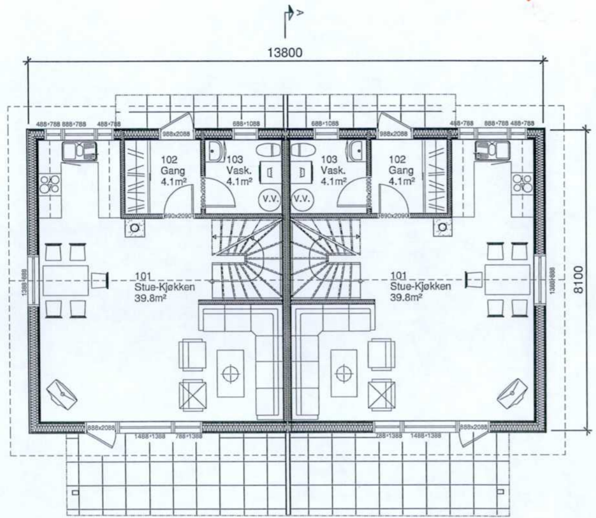
Plan 1. etg.
