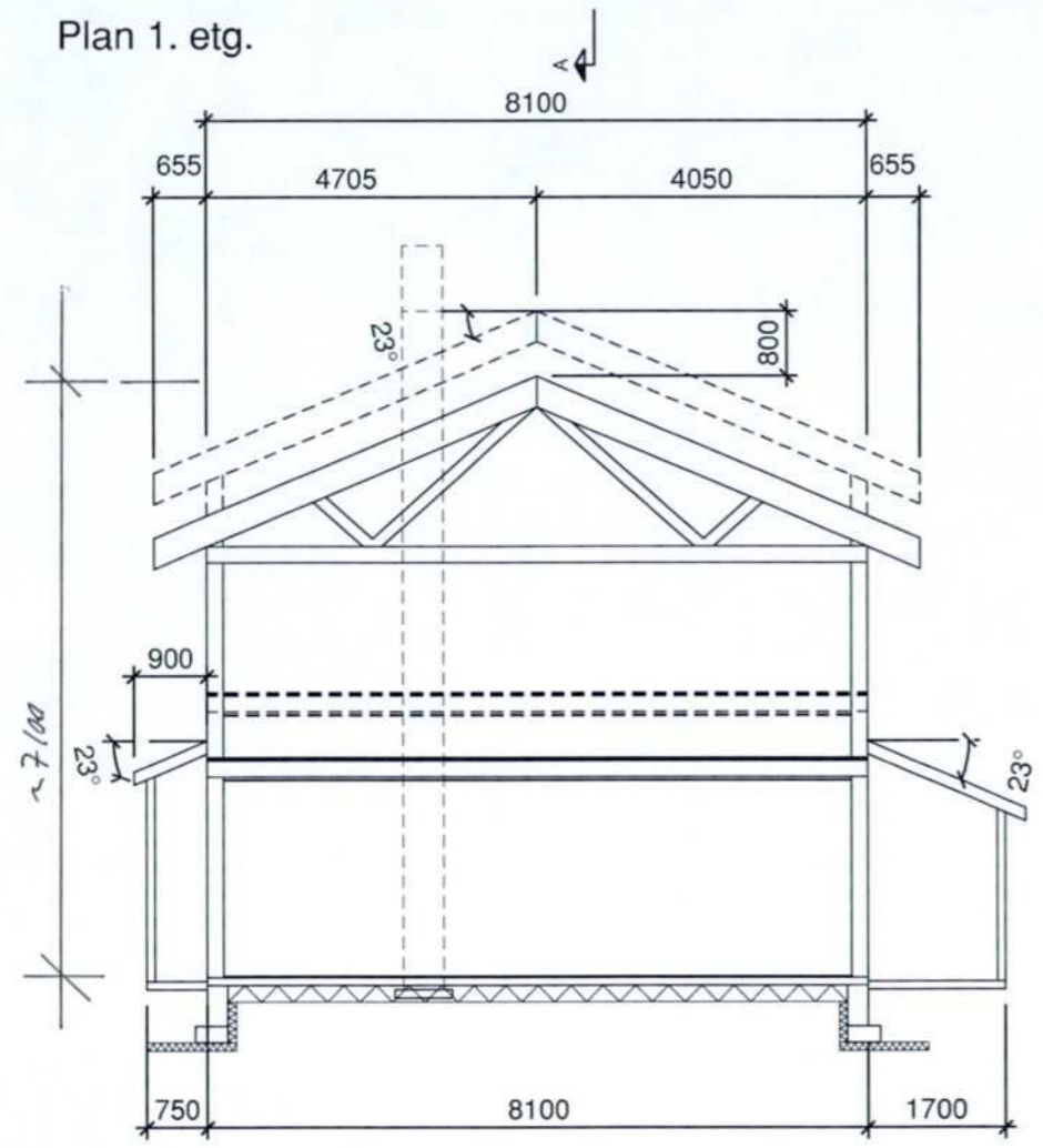
Snitt A-A
