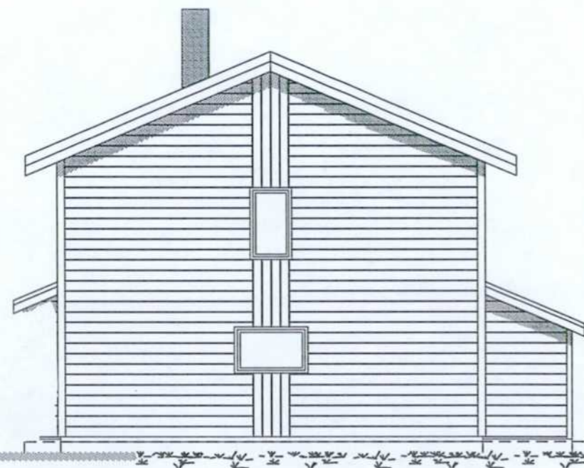
Fasade Øst
