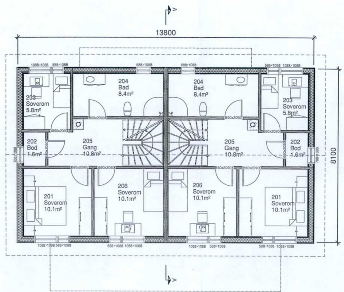
Plan 2. etg.
