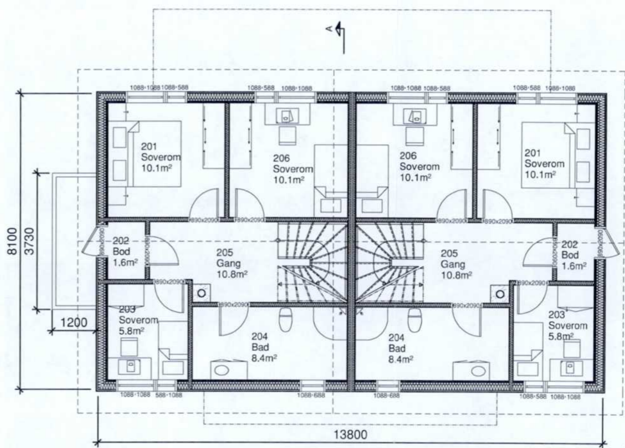
Plan 2. etg.
