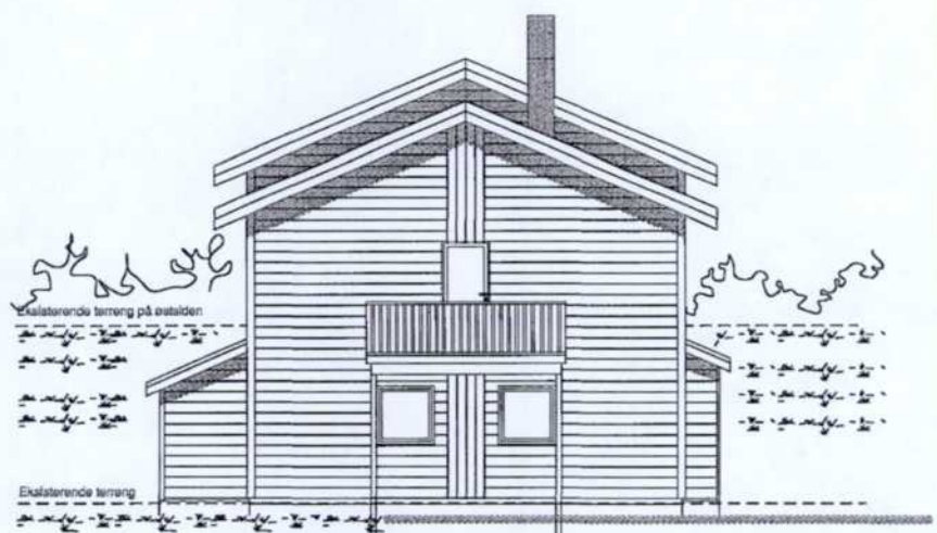
Fasade Vest
