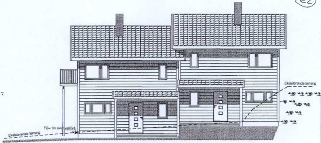
Fasade Syd
