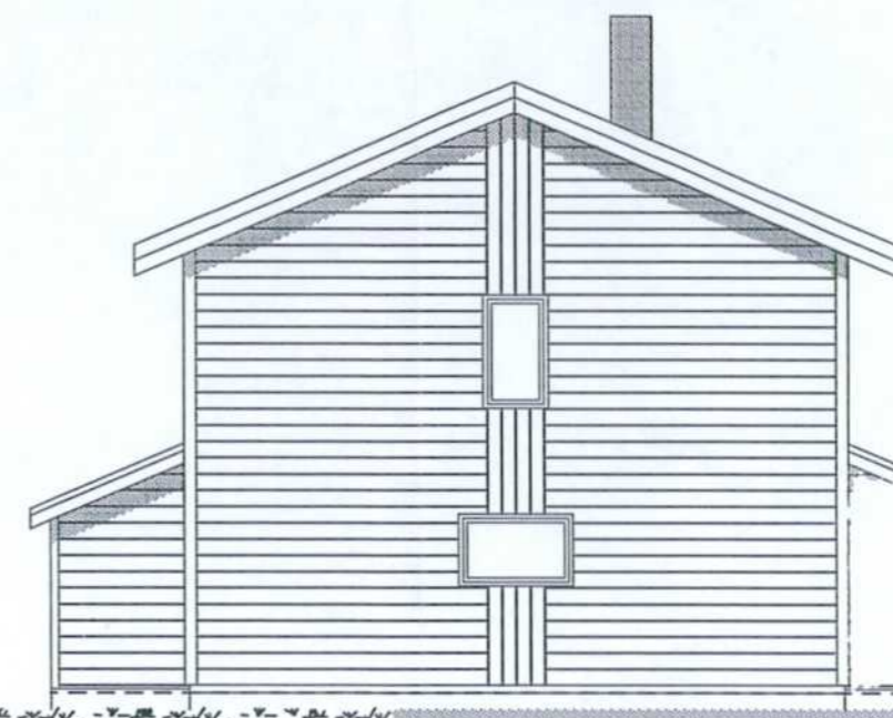
Fasade Vest
