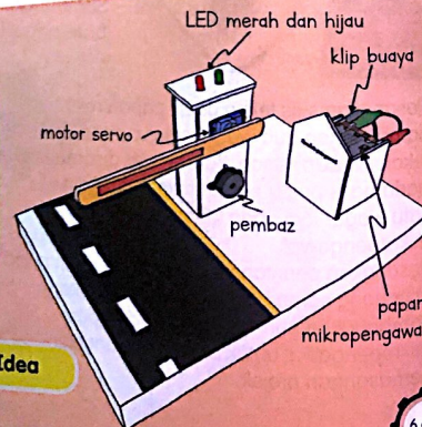
Litar Bergambar Pagar Keselamatan
