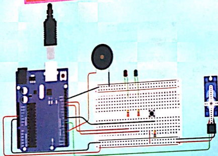
Litar Bergambar Pagar Keselamatan
