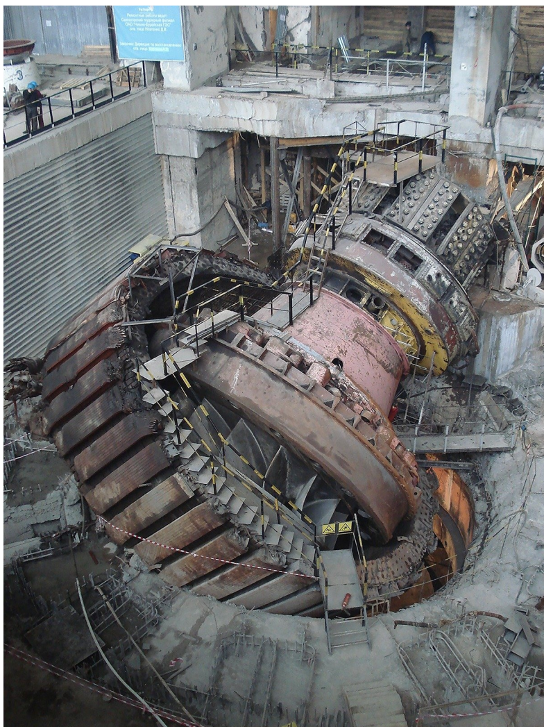
После катастрофы на Саяно-Шушенской ГЭС. В машзале. Фото: Алексей Тарасов / «Новая газета»
