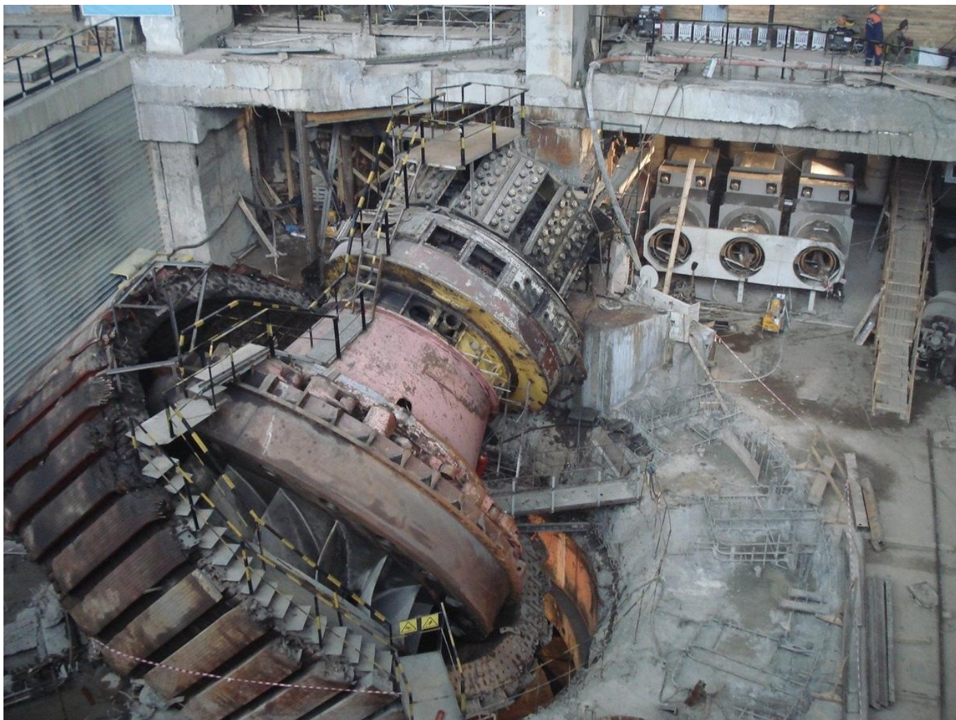
Саяно-Шушенская ГЭС после катастрофы. Ликвидация последствий. Машинный зал. Фото: Алексей Тарасов / «Новая газета»
