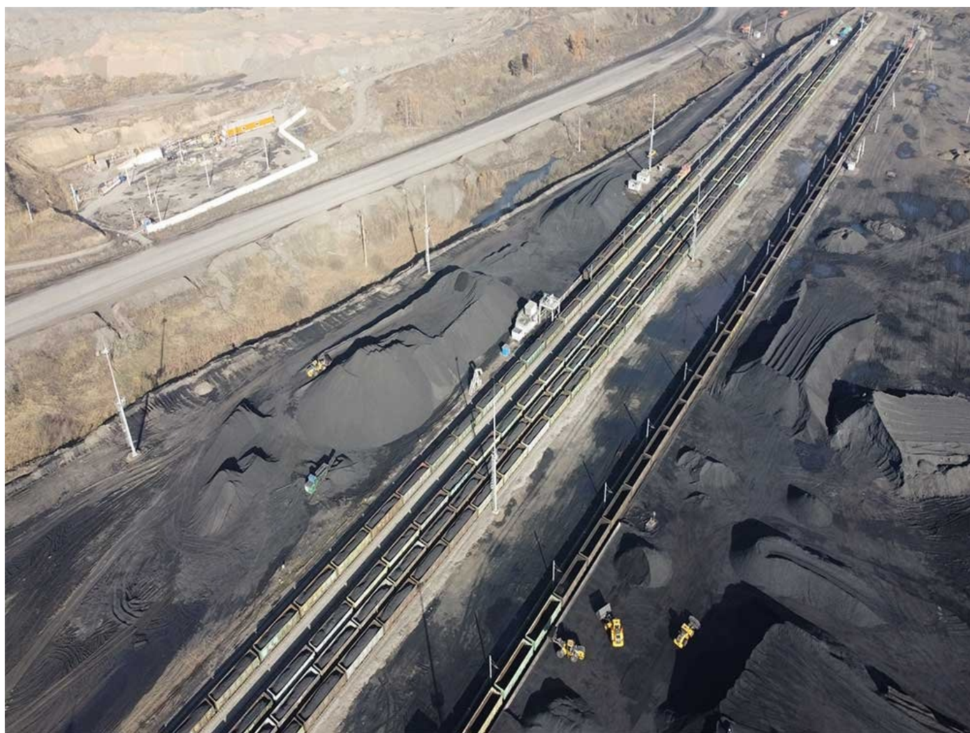
Работы в разрезе «Южный». Фото: Разрез «Южный»
