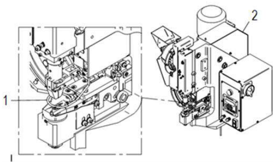
Figura 10: Máquina automática de aplicar ilhós, rebites e adornos - detalhe da vista frontal
