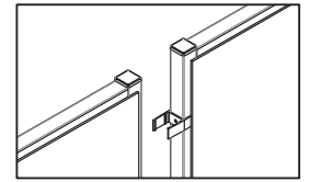
Deux panneaux 180° Utilisez une paire de connecteurs rapides
