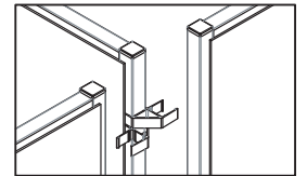
Trois panneaux Utilisez deux paires de connecteurs rapides de coin
