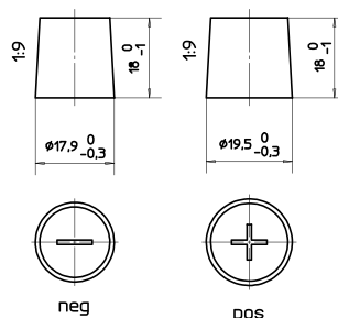
Anschlusspole 1
