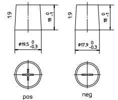
Anschlusspole 1
