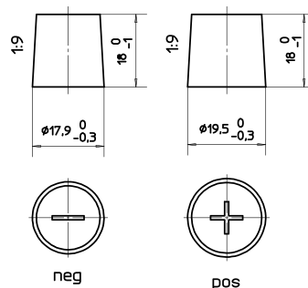
Anschlusspole 1
