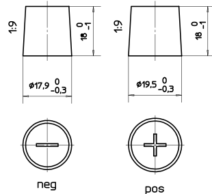
Anschlusspole 1
