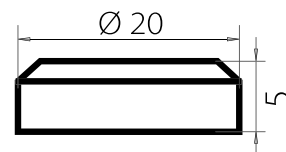
Anschlusspole T5
