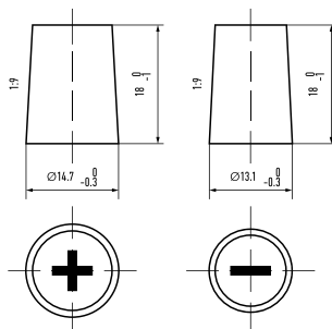
Anschlusspole 3
