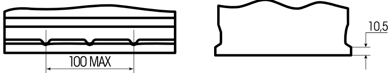
Bodenleiste B01
