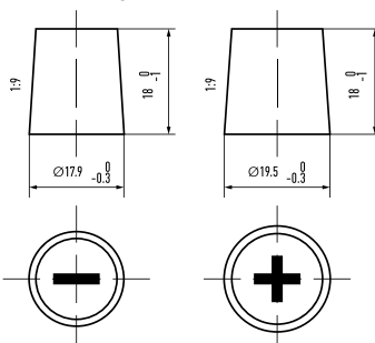
Anschlusspole 1
