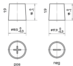
Anschlusspole 1
